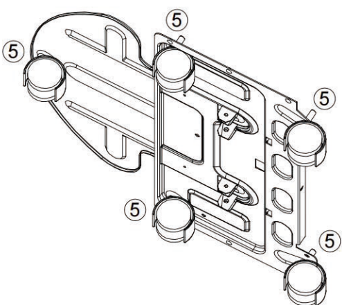
5: Monter 5 hjul på bunnpanelet 5x E
