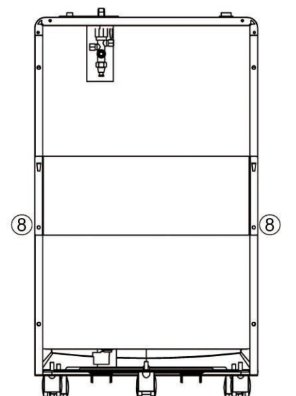
8: Monter bakpanel på sidepanelene 2x B
